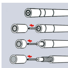
Třístupňové odizolování koaxiálního kabelu
